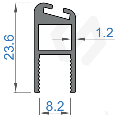
Sistem Kodu 4809 Ağırlık (kg/mt) 0,250
