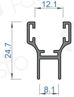
Sistem Kodu 4806 Ağırlık (kg/mt) 0,227
