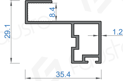
Sistem Kodu 5196 Ağırlık (kg/mt) 0,358
