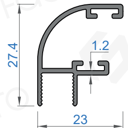
Sistem Kodu 11003 Ağırlık (kg/mt) 0,272
