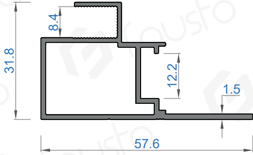
Sistem Kodu 5195 Ağırlık (kg/mt) 0,558
