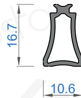
Sistem Kodu 1661 Ağırlık (kg/mt) 0,142
