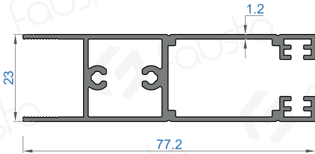
Sistem Kodu 1659 Ağırlık (kg/mt) 0,903
