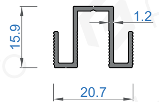
Sistem Kodu 1660 Ağırlık (kg/mt) 0,205
