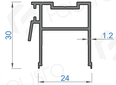
Sistem Kodu 1658 Ağırlık (kg/mt) 0,401
