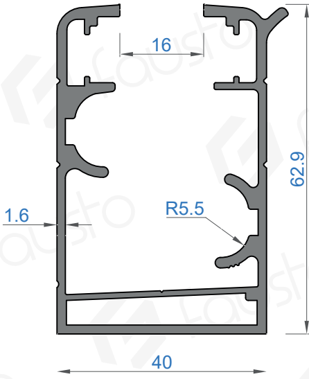
Sistem Kodu 1611 Ağırlık (kg/mt) 1,325
