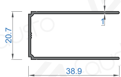
Sistem Kodu 50112 Ağırlık (kg/mt) 0,261
