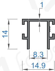
Sistem Kodu 50110 Ağırlık (kg/mt) 0,138
