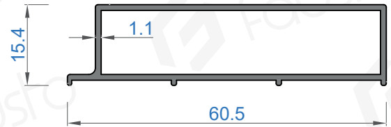
Sistem Kodu 50109 Ağırlık (kg/mt) 0,428
