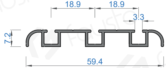
Sistem Kodu 50107 Ağırlık (kg/mt) 0,333
