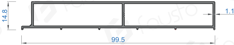
Sistem Kodu 50108 Ağırlık (kg/mt) 0,691
