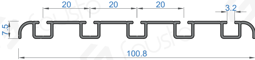
Sistem Kodu 50106 Ağırlık (kg/mt) 0,552
