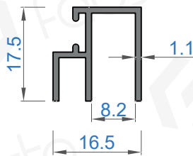
Sistem Kodu 50111 Ağırlık (kg/mt) 0,185
