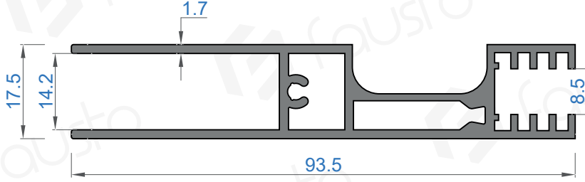
Sistem Kodu 50104 Ağırlık (kg/mt) 1,158
