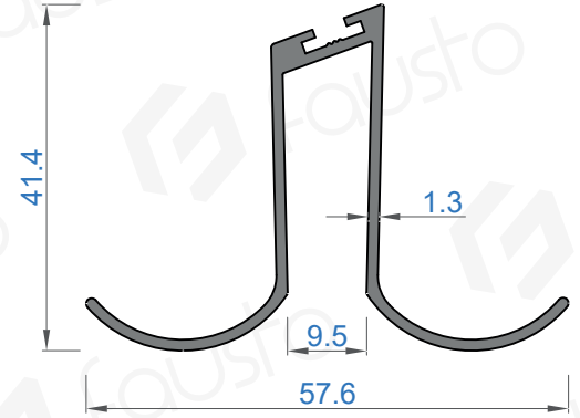
Sistem Kodu 50105 Ağırlık (kg/mt) 0,494
